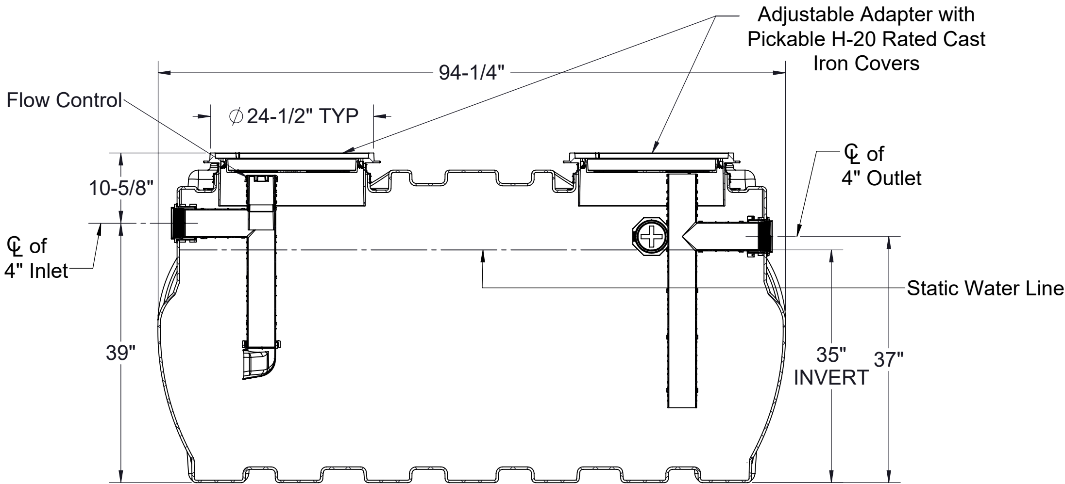
SECTION A-A
