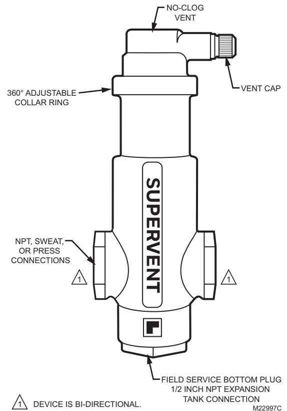
Fig. 1. SuperVent
